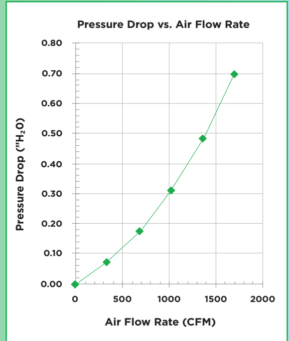
(based on 16x20x4 M15 mini pleat)
